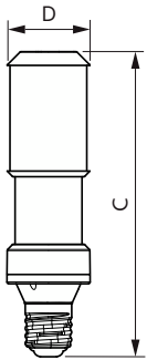
MAS LED SON-T IF 12Klm 65W 740 E40
